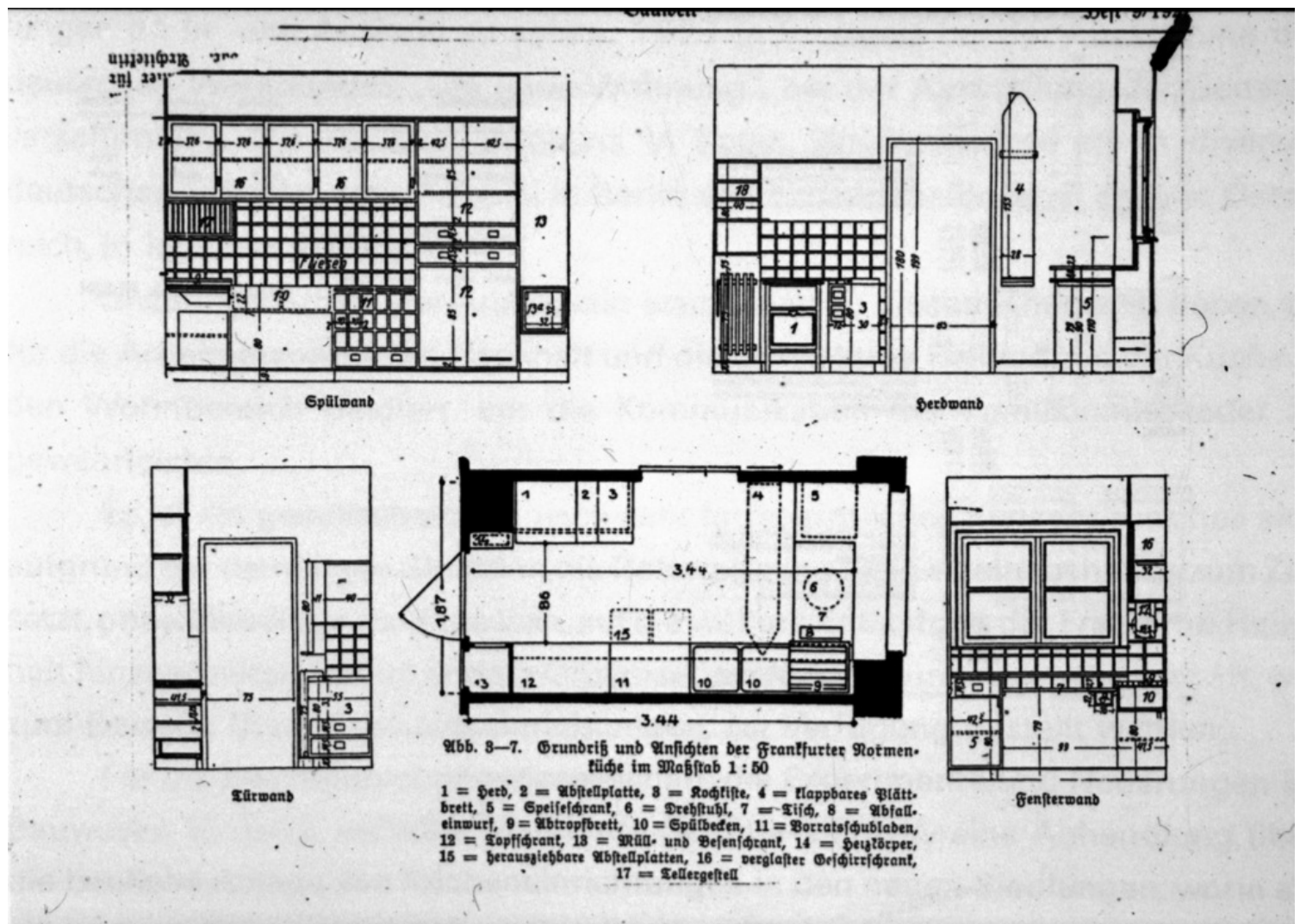
(εικ.2). Margarete Schütte-Lihotzky, σχέδιο για την κουζίνα της Φρανκφούρτης, δεκαετία 1920. (Πηγή : http://www.hiddenarchitecture.net/2017/11/frankfurt-kitchen.html )
