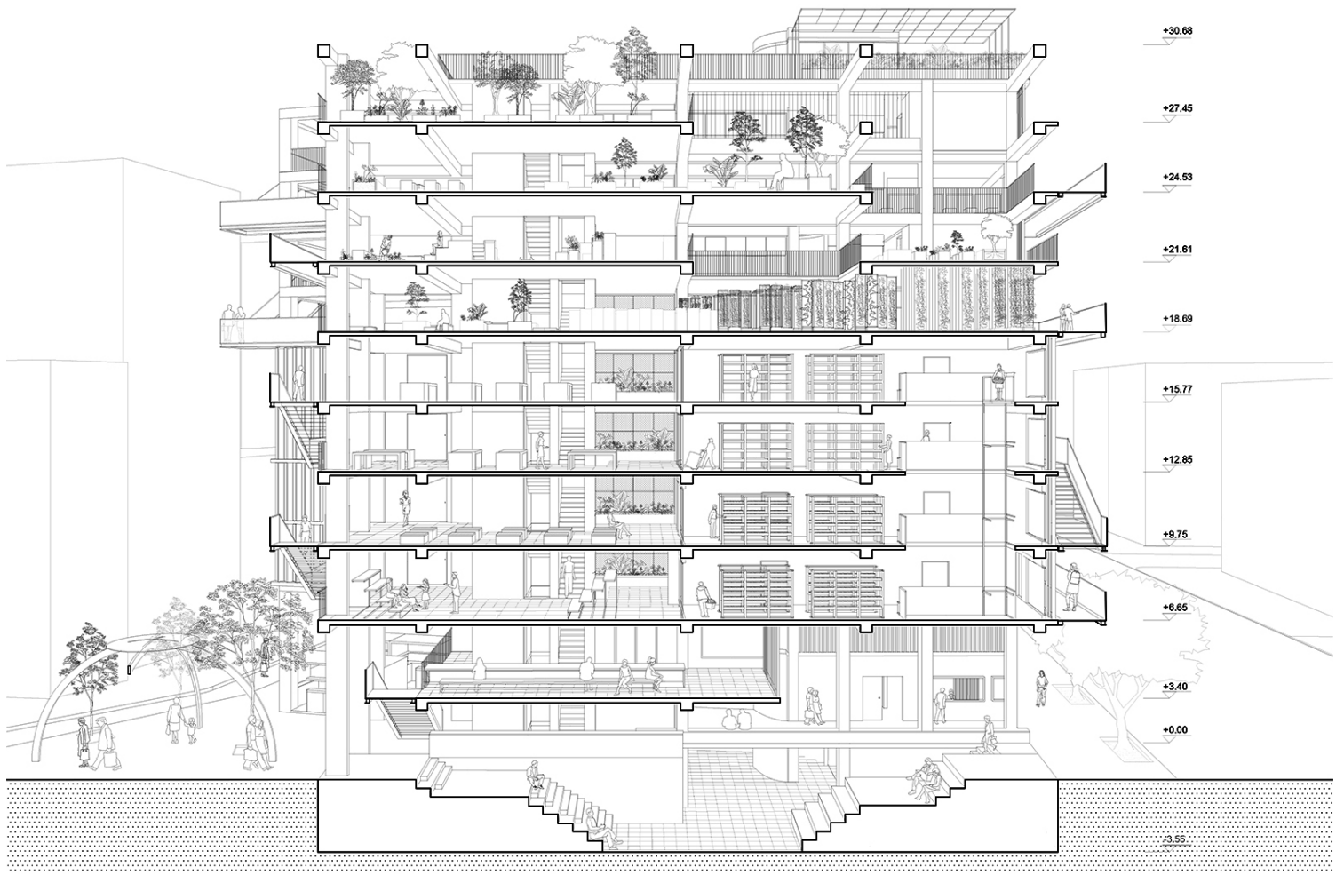
SECTION A-A'
