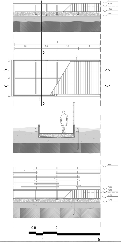
ΣΑΝΙΔΕΣ 12x3
