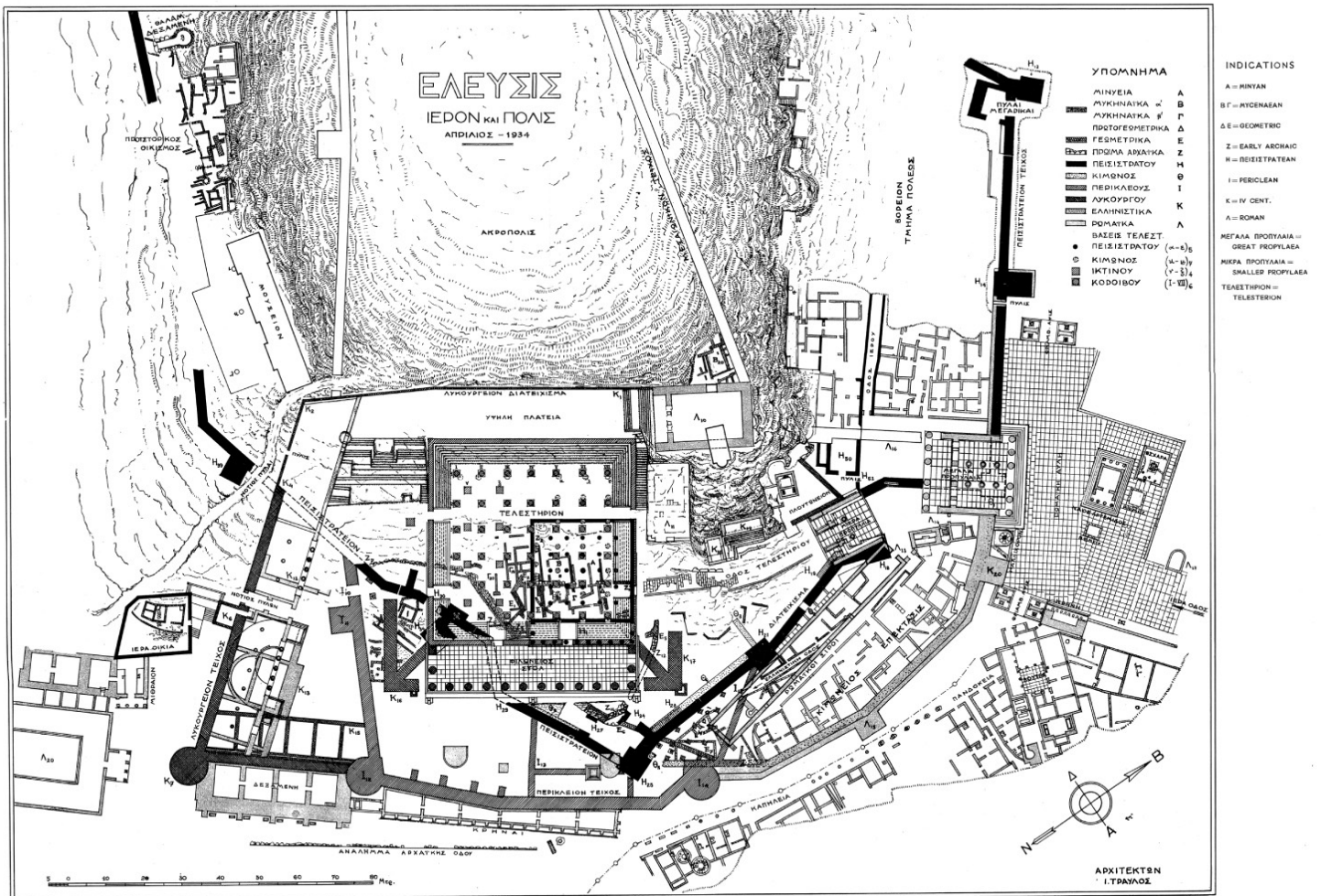
Ι. Τραυλός, πρώτο τοπογραφικό σχέδιο για την πόλη και το ιερό της Ελευσίνας, 1934.
