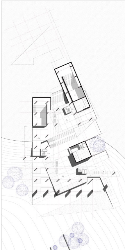
ΑΙΘΟΥΣΕΣ ΘΕΩΡΙΑΣ - ΑΜΦΙΘΕΑΤΡΑ (+7.90) 8. Ημιλιπαθρία Γλαστέα 9. Μικρή Γλαστέα 10. Κώλακιο 11. Αίθουσα Θεωρίας - Μεγάλο Αμφιθέατρο
