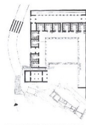
Ιερό της Αρτέμιδος στη Βρουαίνα διόδρομος | δωμάτια | στοά | αίθριο
