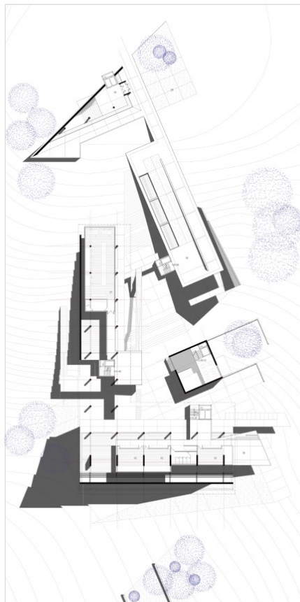
ΠΑΤΑΡΙ ΣΥΝΟΛΩΝ - ΒΙΒΛΙΟΘΗΚΗ (+15.40) 15. Αίθουσα Συνόλων 16. Υπεράθριο Θεατρικό 17. Βιβλιοθήκη Αρχείο 18. Φοιτημένο Δάμα 19. Φοιτημέ Αίθουσα Εκδηλώσεων 20. Βιβλιοθήκη - Αρχείο
