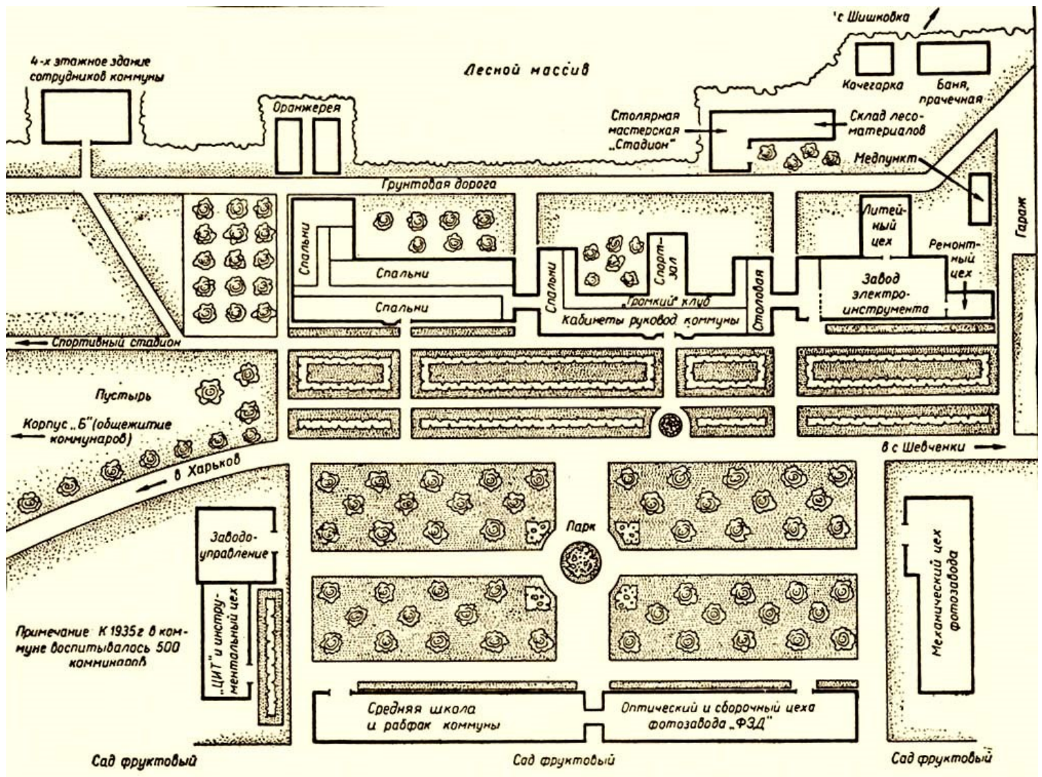
Εικόνα 2. Σχηματική κάτοψη της κομμούνας στο Χάρκοβο, καθώς δεν υπάρχουν αεροφωτογραφίες και πολλά από τα κτήριά της πλέον δεν σώζονται ύστερα από τις καταστροφές του Β' Παγκοσμίου Πολέμου. Στο πάνω μέρος του σχήματος βρίσκονται τα κτήρια κατοίκησης, στη μέση πάρκο και άλσος και στο κάτω μέρος βρίσκεται το σχολείο και το εργοστάσιο φωτογραφικών μηχανών.
