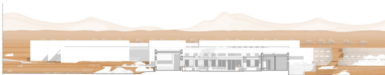
ΤΟΜΗ Δ-Δ ΚΑΙΜΑΚΑ 1 | 150
